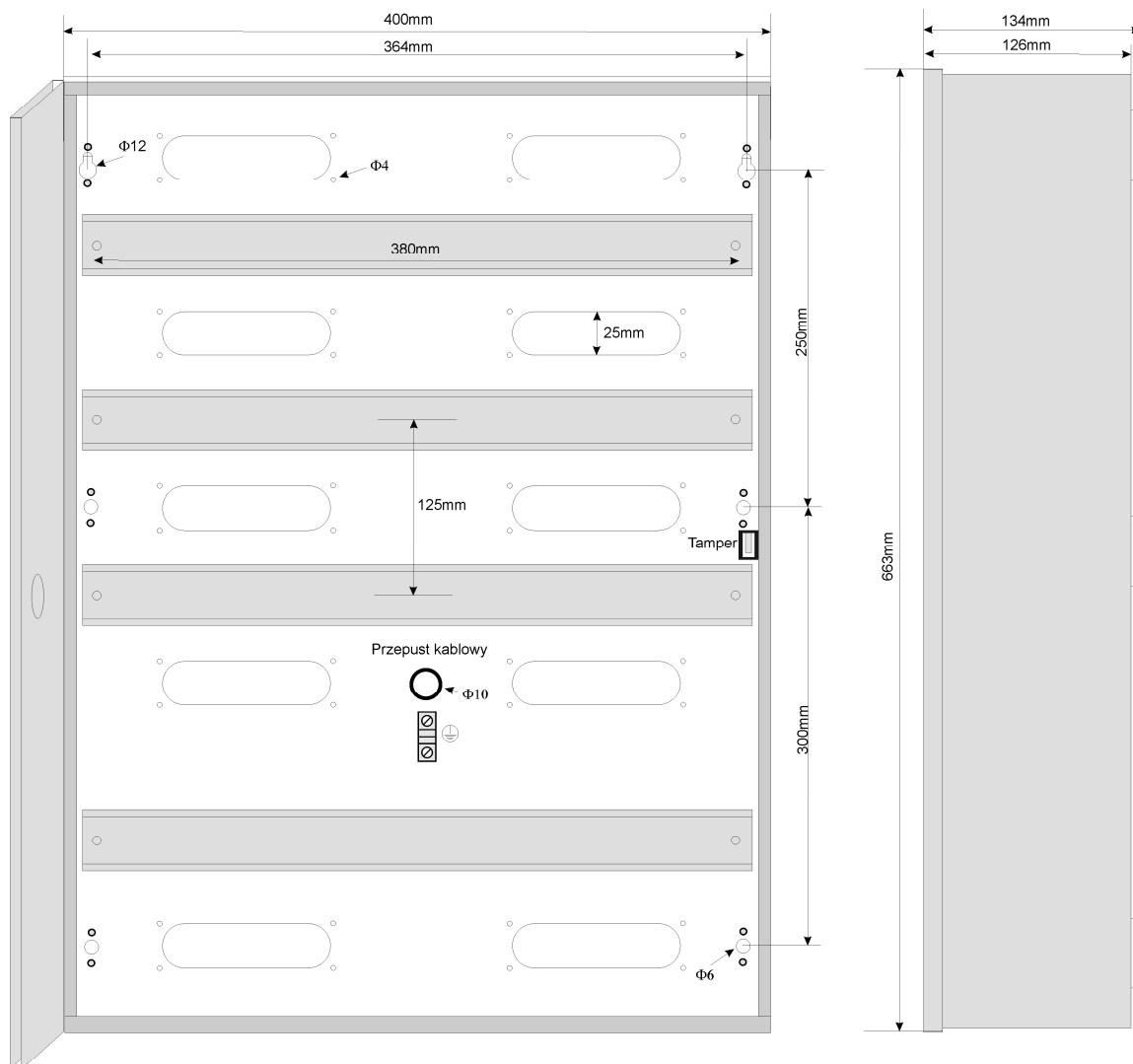
Rys. 1 Widok wnętrza obudowy ME-5
